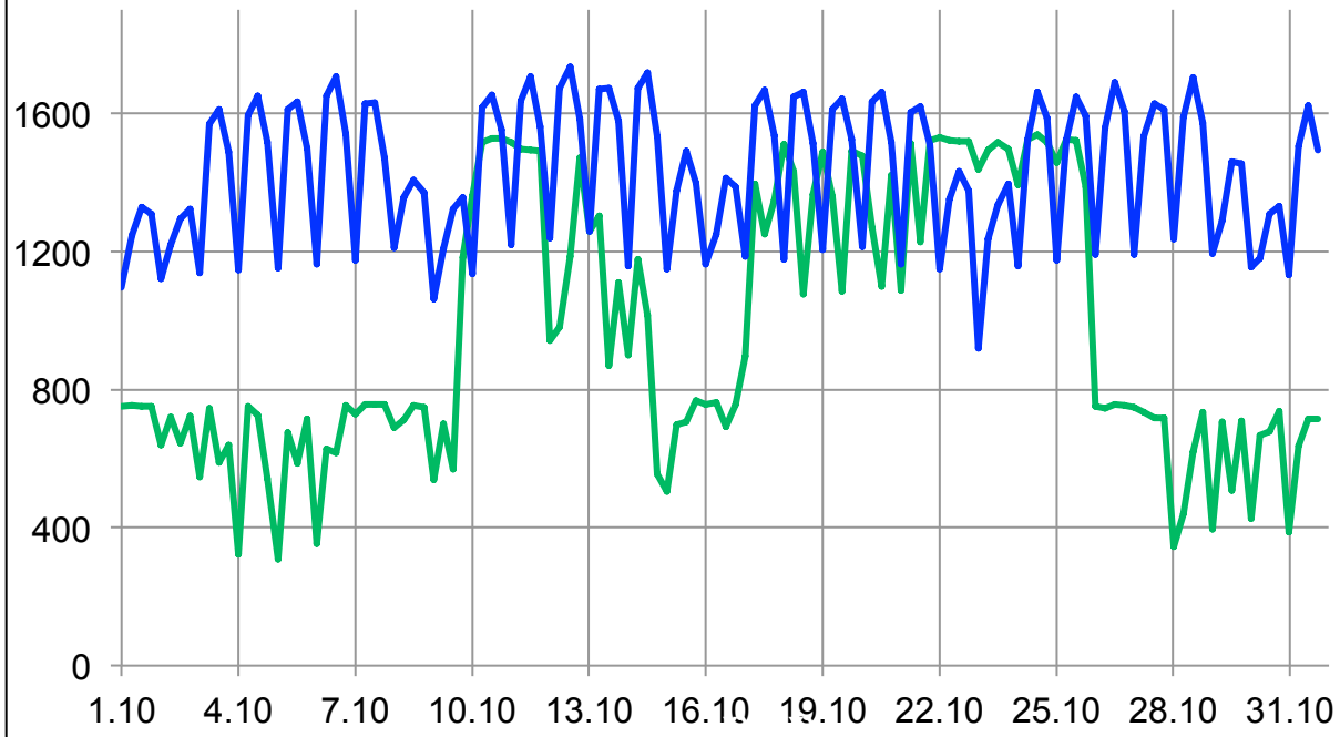
Hamburger Strombedarf (blau) und Einspeisung des Kraftwerks Moorburg (grün) im Oktober 2016 (in MW)
