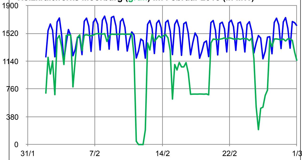
Hamburger Strombedarf (blau) und Einspeisung des Heizkraftwerks Moorburg (grün) im Februar 2018 (in MW)
