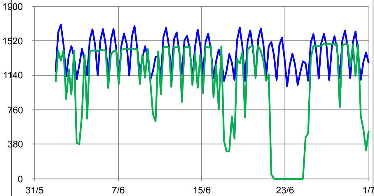
Hamburger Strombedarf (blau) und Einspeisung des Heizkraftwerks Moorburg (grün) im Juni 2018 (in MW)
