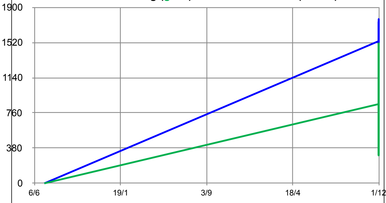
Hamburger Strombedarf (blau) und Einspeisung des Heizkraftwerks Moorburg (grün) im November 2018 (in MW)
