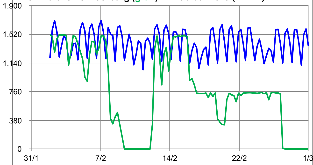
Hamburger Strombedarf (blau) und Einspeisung des Heizkraftwerks Moorburg (grün) im Februar 2019 (in MW)
