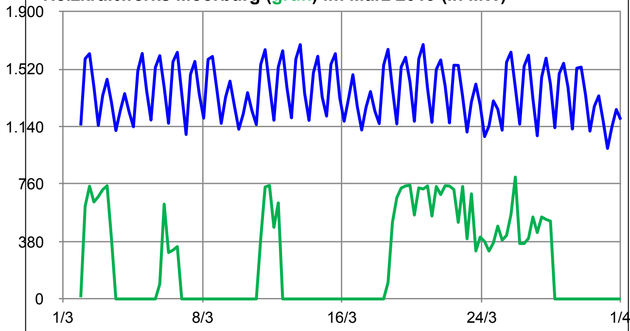
Hamburger Strombedarf (blau) und Einspeisung des Heizkraftwerks Moorburg (grün) im März 2019 (in MW)
