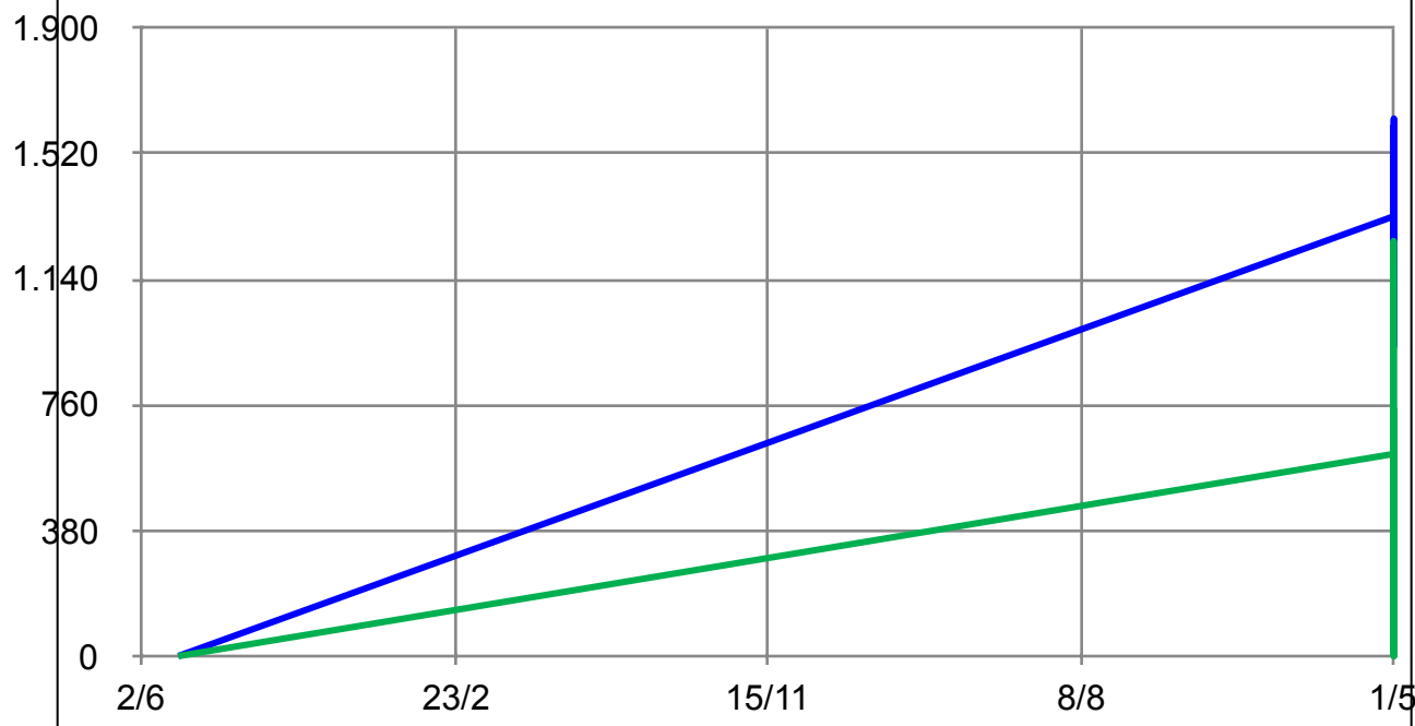
Hamburger Strombedarf (blau) und Einspeisung des Heizkraftwerks Moorburg (grün) im April 2019 (in MW)
