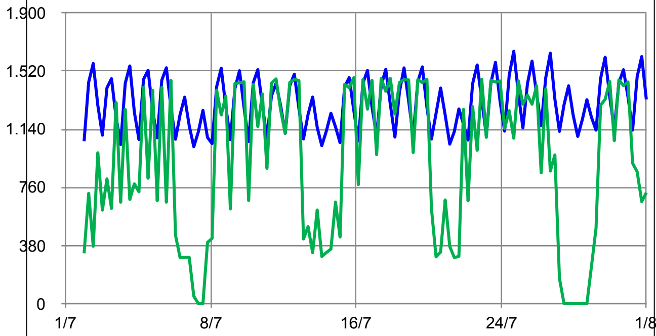
Hamburger Strombedarf (blau) und Einspeisung des Heizkraftwerks Moorburg (grün) im Juli 2019 (in MW)
