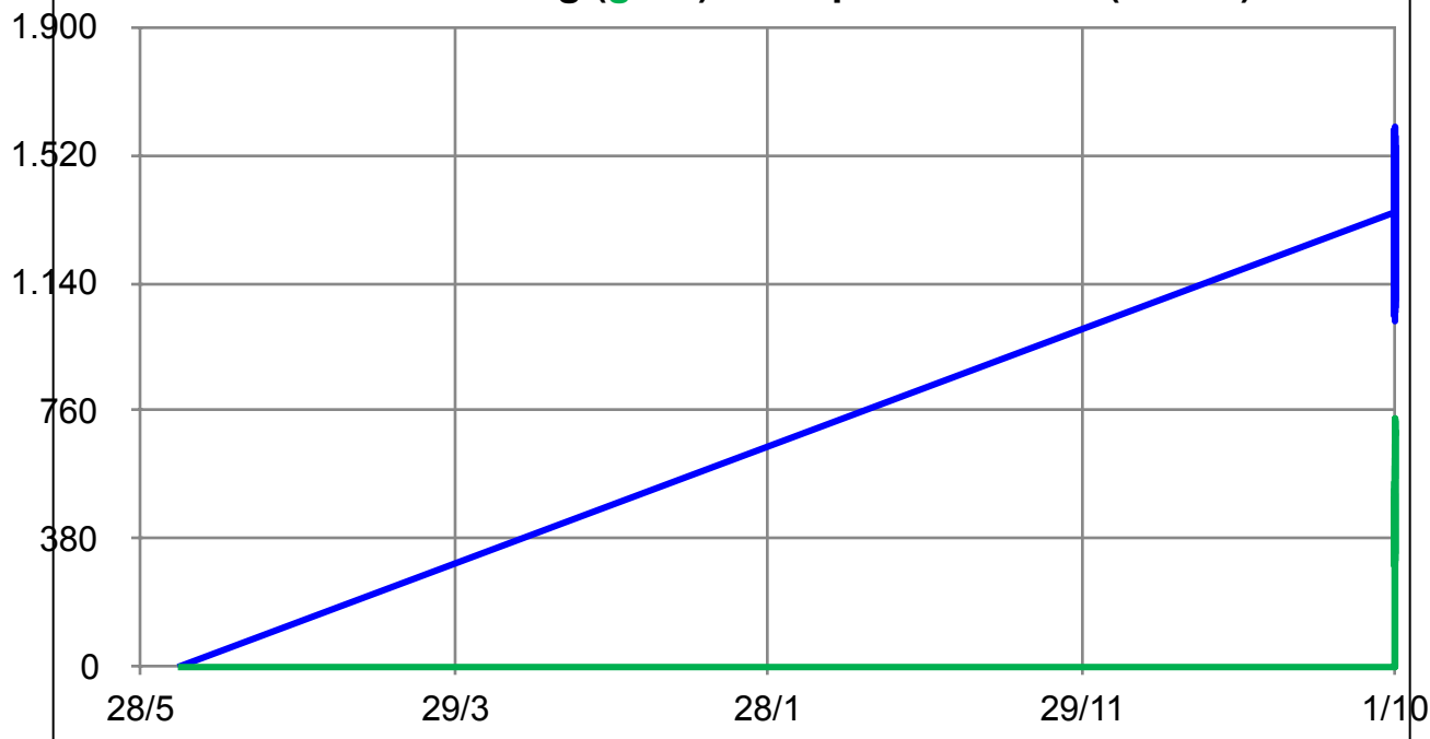
Hamburger Strombedarf (blau) und Einspeisung des Heizkraftwerks Moorburg (grün) im September 2019 (in MW)
