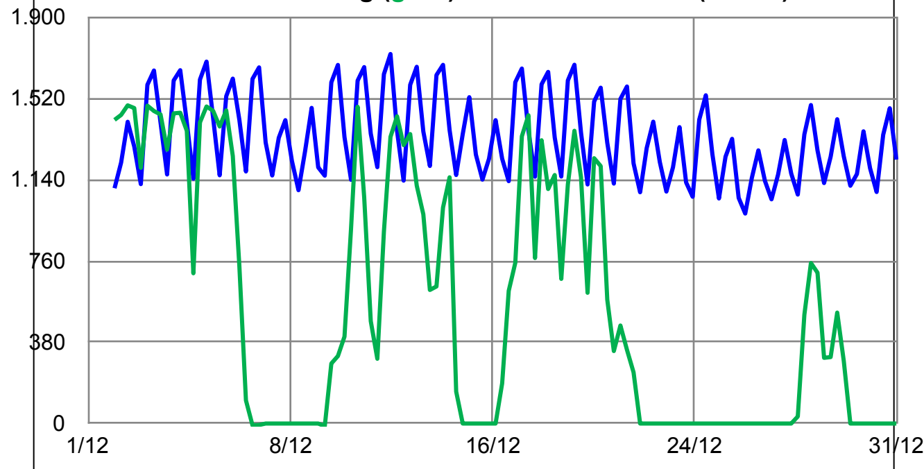
Hamburger Strombedarf (blau) und Einspeisung des Heizkraftwerks Moorburg (grün) im Dezember 2019 (in MW)
