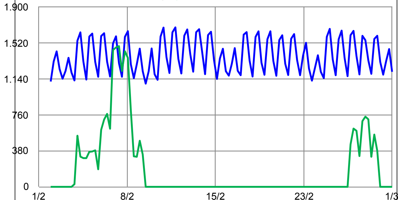
Hamburger Strombedarf (blau) und Einspeisung des Heizkraftwerks Moorburg (grün) im Februar 2020 (in MW)
