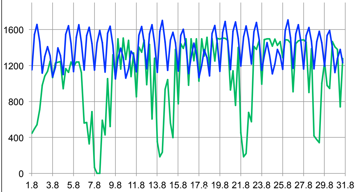
Hamburger Strombedarf (blau) und Einspeisung des Kraftwerks Moorburg (grün) im August 2016 (in MW)
